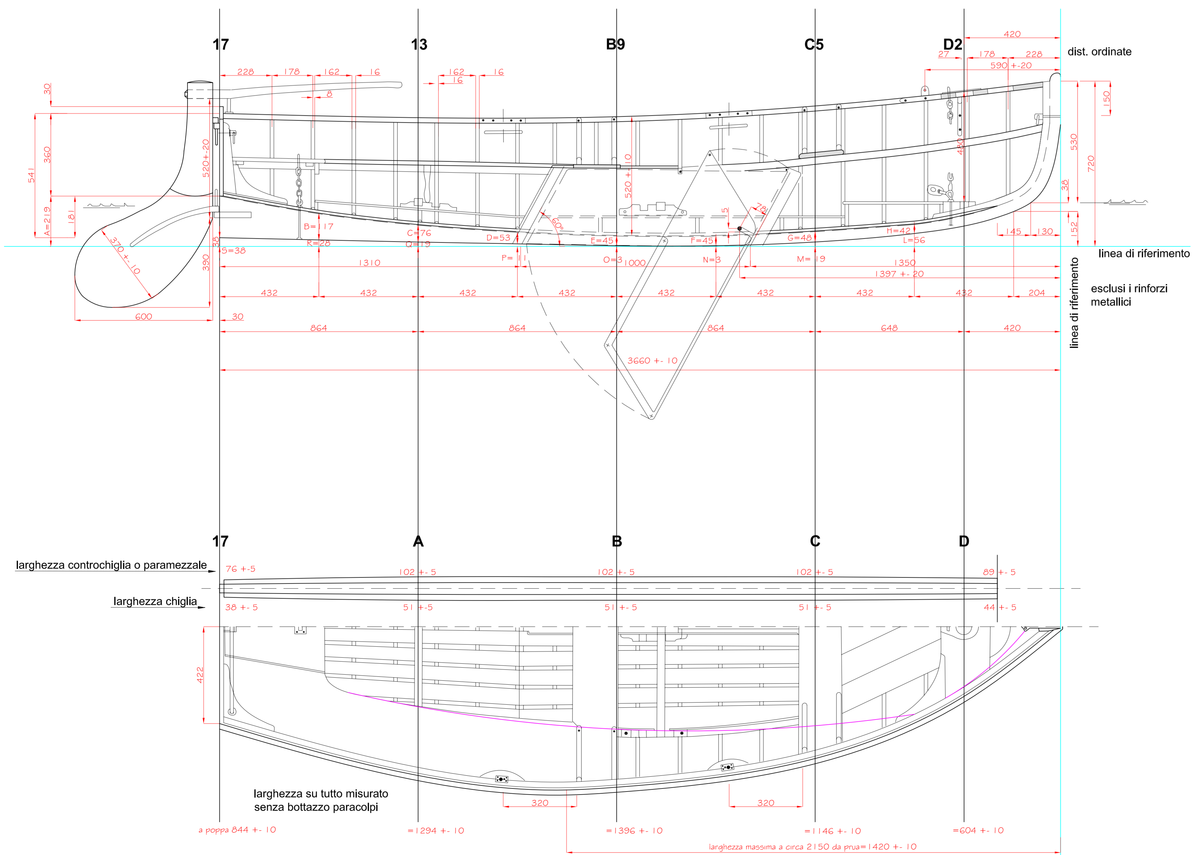
SCAFO - vista dall'alto
