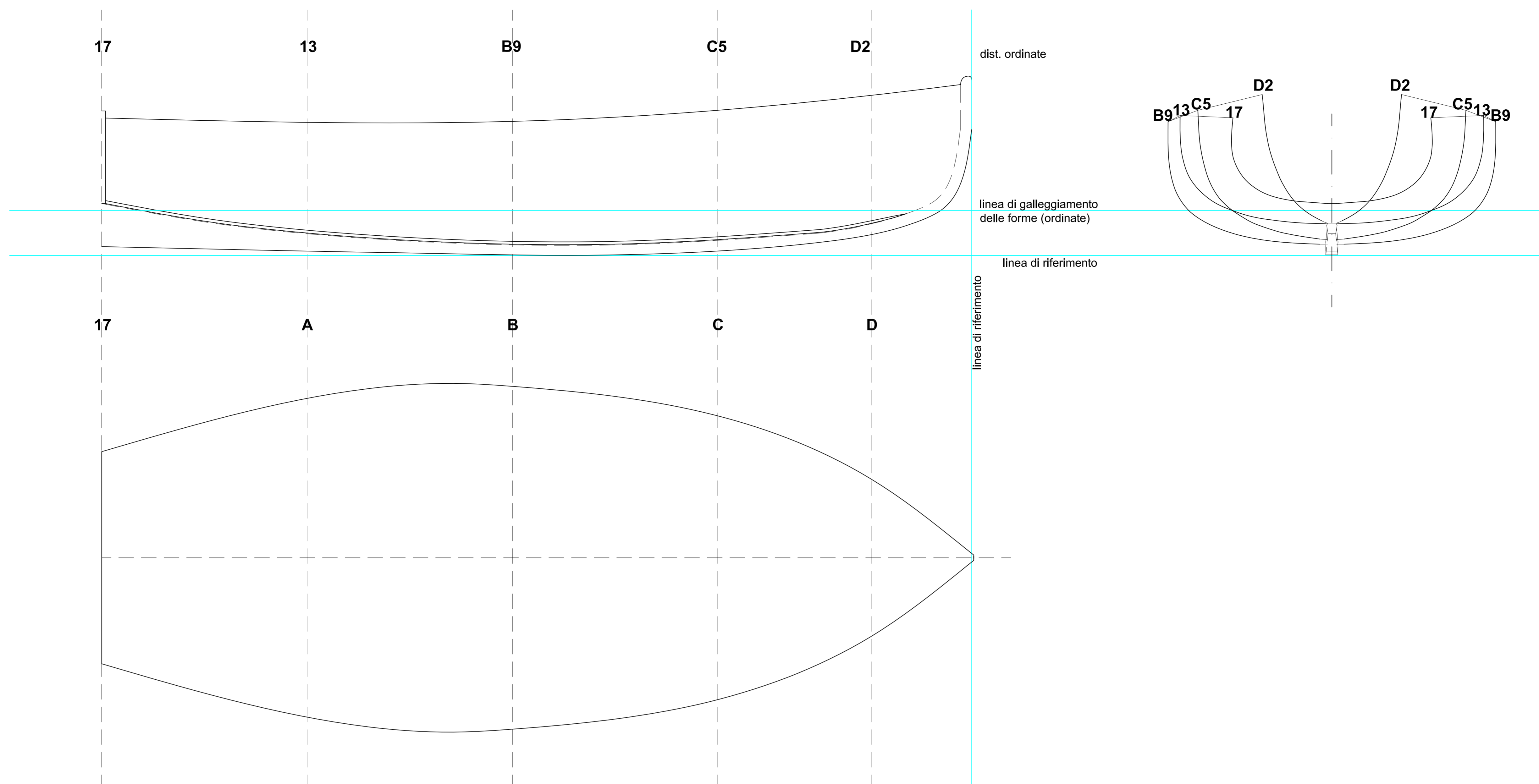
SCAFO - sezione longitudinale (Tolleranza sulle misure da A ad S +/- 10)
